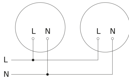
aansluitschema master/master Bluetooth
